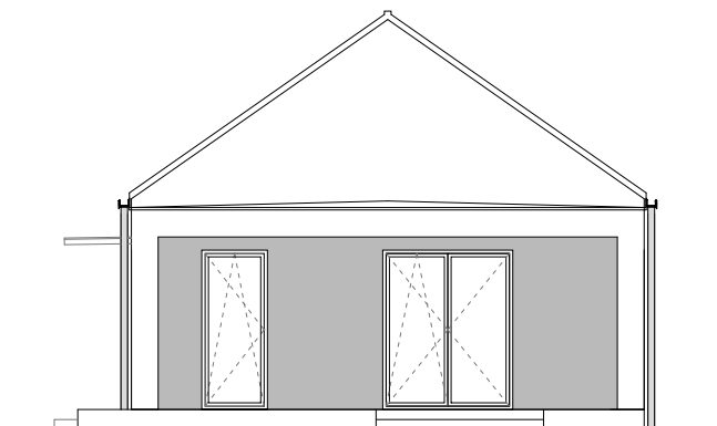
ELEWACJA BOCZNA 2
