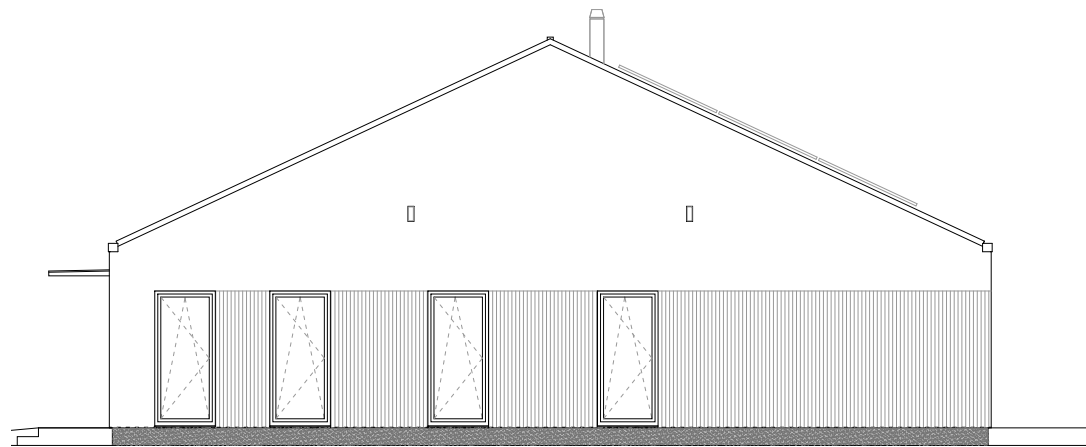
ELEWACJA BOCZNA 1
