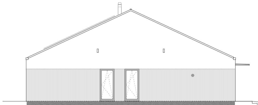
ELEWACJA BOCZNA 2
