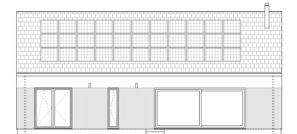
ELEWACJA OGRODOWA
