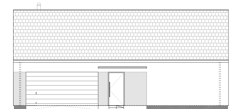
ELEWACJA FRONTOWA
