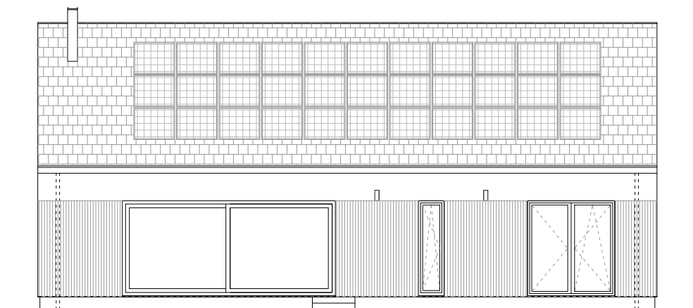
ELEWACJA OGRODOWA
